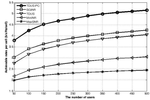
그림 4. K=4, \text{SNR}=10\text{dB} 일 때 다중 셀 상향링크 네트워크의 사용자 수에 따른 데이터 전송률 Fig. 4 Achievable data rates of the proposed algorithm in multi-cell networks for varying number of users in a cell for K=4 and \text{SNR}=10\text{dB}
