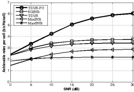
그림 1. K=3, N=100 일 때 다중 셀 상향링크 네트워크의 SNR에 따른 데이터 전송률 Fig. 1 Achievable data rate of the proposed algorithm in uplink multi-cell networks for varying SNRs for K=3 and N=100
