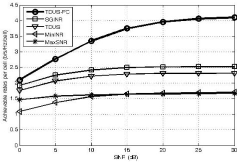
그림 2. K=4, N=100 일 때 다중 셀 상향링크 네트워크의 SNR에 따른 데이터 전송률 Fig. 2 Achievable data rates of the proposed algorithm in uplink multi-cell networks for varying SNRs for K=4 and N=100
