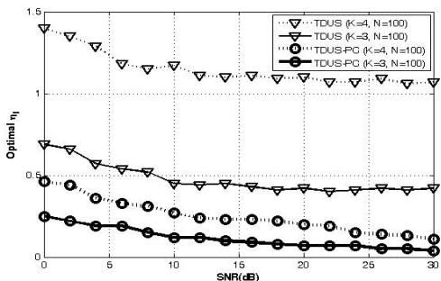
그림 3. 그림 1과 그림 2의 TDUS 기술과 TDUS-PC 기술의 SNR에 최적의 간섭 임계값 \eta_I Fig. 3 The optimal \eta_I of TDUS and TDUS-PC scheme for varying SNRs in Fig.1 and Fig.2
